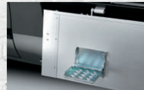
KIPPBARE TRITTBRETTER AUF DER INNENSEITE DER PRITSCHENWAND
